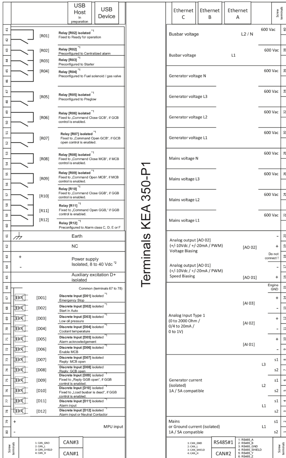
Abb. 6: Anschlussplan KEA 350 RP-P1 / KEA 350 P1 (-LT)
